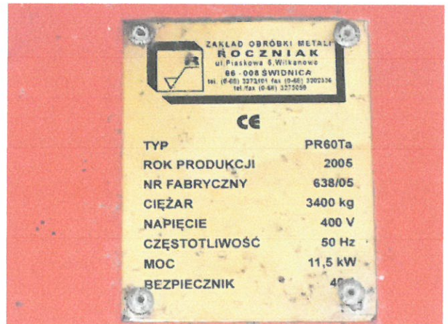
Fot. Nr 7 – tabliczka znamionowa;
