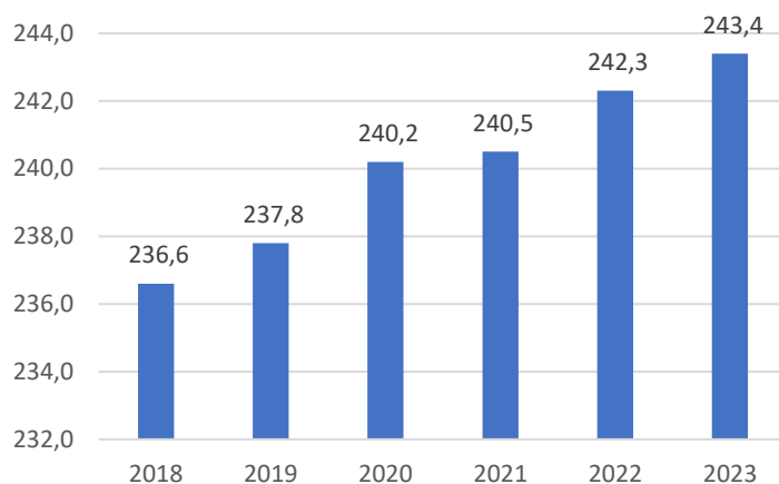
Wykres 9. Długość czynnej sieci rozdzielczej – wodociąg.
